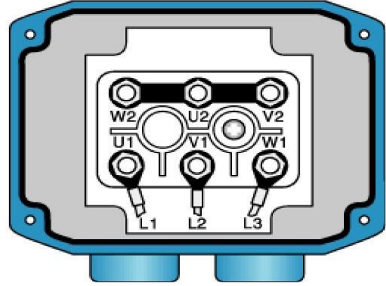
YILDIZ BAĞLANTI
