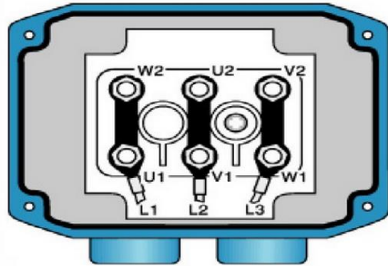
ÜÇGEN BAĞLANTI
