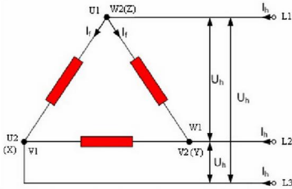
ÜÇGEN BAĞLANTI
