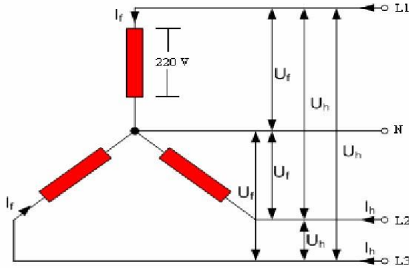
YILDIZ BAĞLANTI
